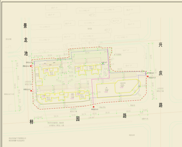
现状总平面图
