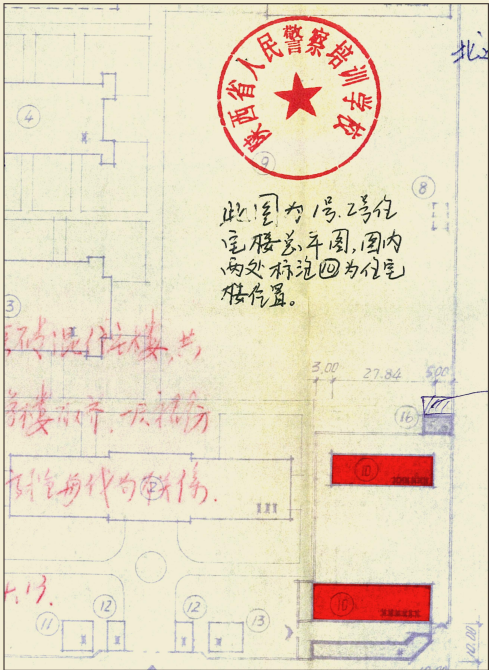
原规划总平图
