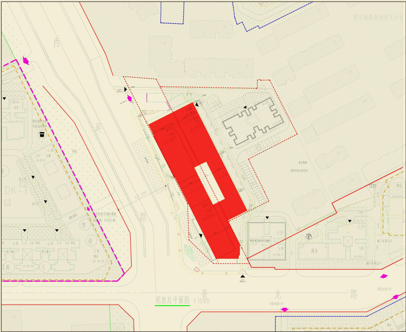
现状总平面图
