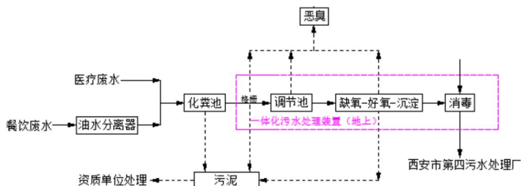
图4 设计废水处理工艺流程图
